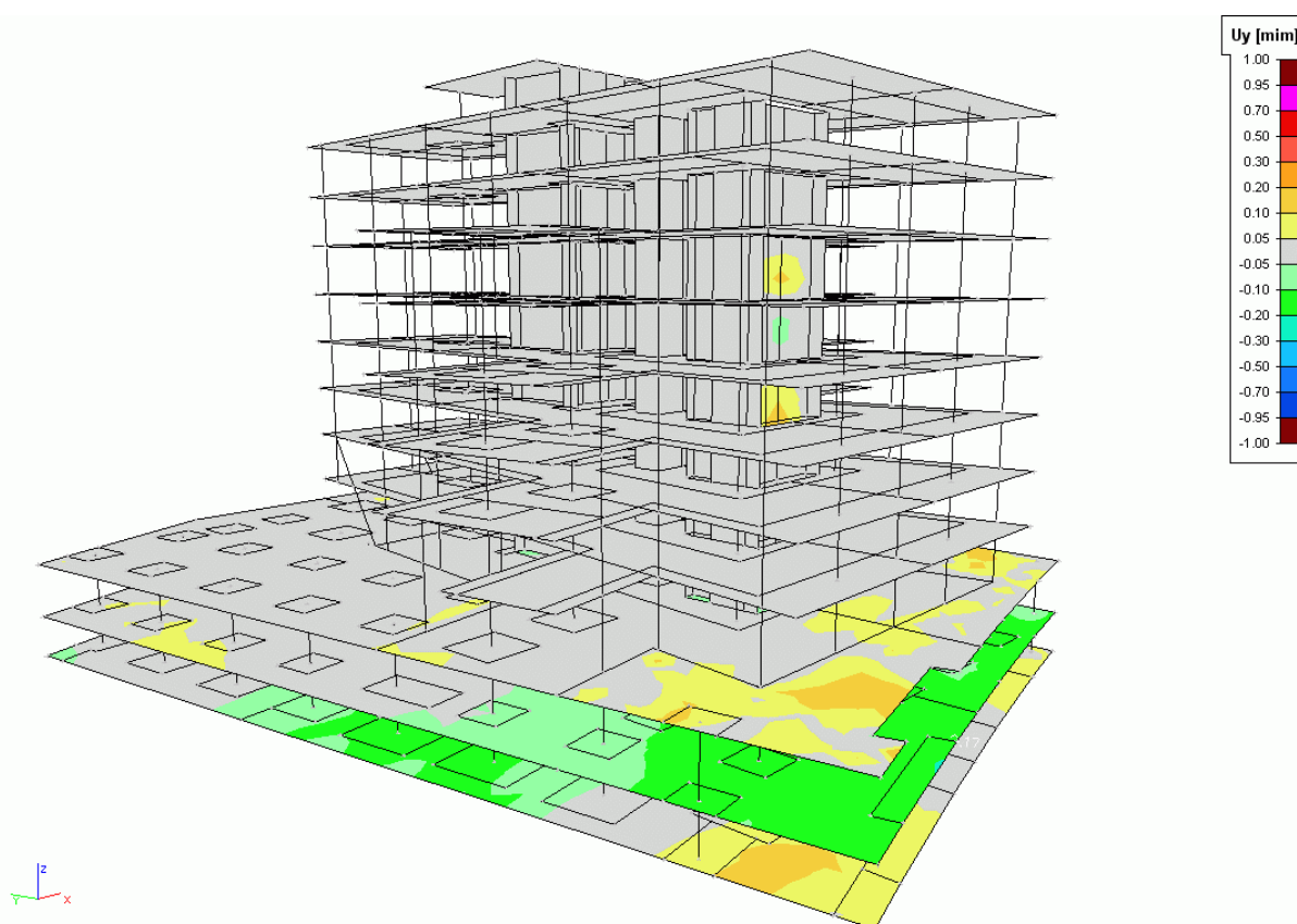
Obr.5 Izolinie normalizovaných horizontálních vibrací stropních desek v časovém kroku 0,144 s při buzení vibracemi od přejezdu vlaku po železnici (normalizováno vůči maximu horizontálního kmitání základové desky rovné 1,0)
