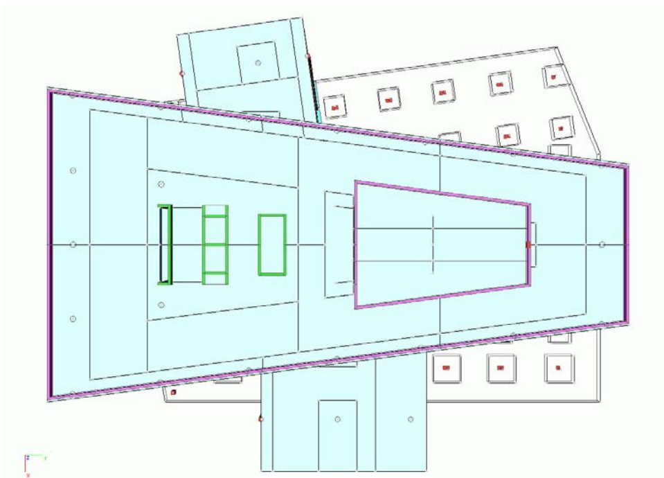
Obr.1 Výpočetní model konstrukce budovy včetně podzemních podlaží a spojovacích krčků;
