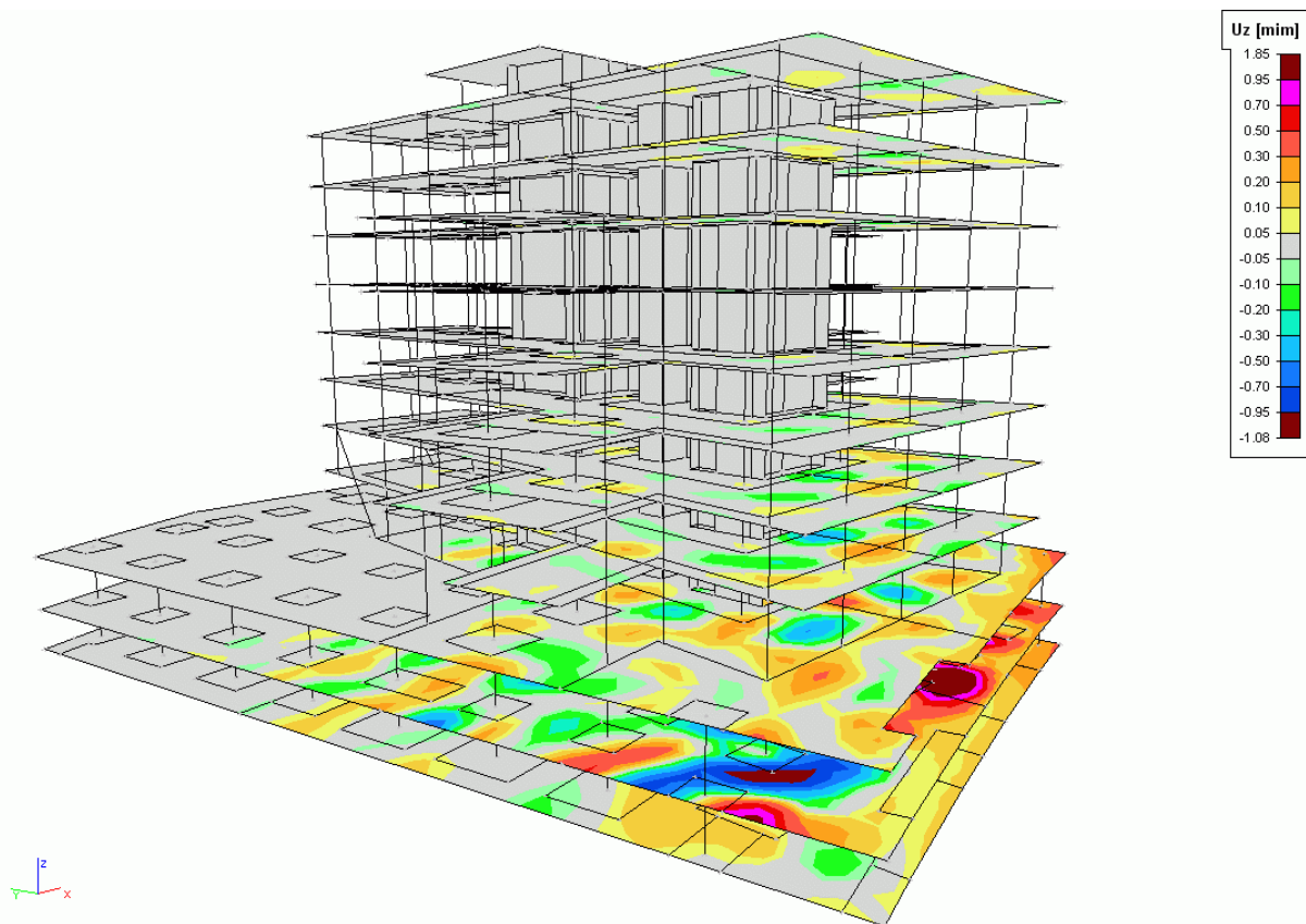
Obr.4 Izolinie normalizovaných vertikálních vibrací stropních desek v časovém kroku 0,114 s při buzení vibracemi od přejezdu vlaku po železnici (normalizováno vůči maximu vertikálního kmitání základové desky rovné 1,0)
